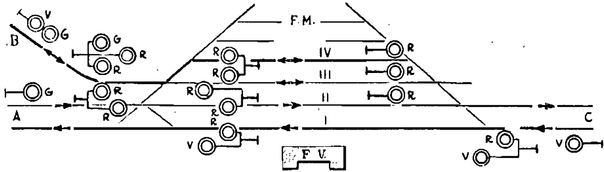
Arrivo da B in IV linea Transito da C ad A
