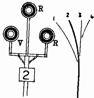
Segnale a candelliere integrato da indicatore a via libera per la direzione 2
