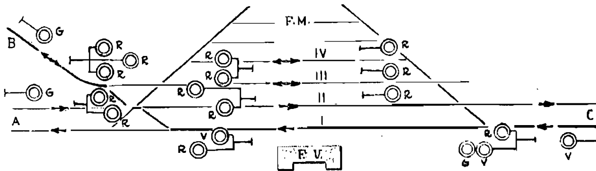
Transito da C a B (attraverso la I linea)
