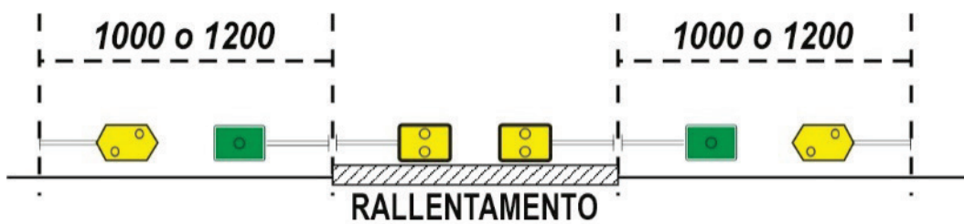
Rallentamento su linea a doppio binario interessando un solo binario
