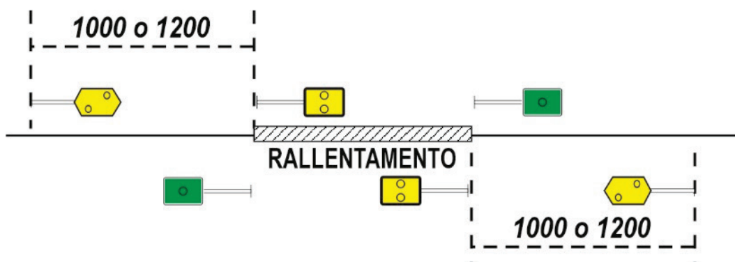
Rallentamento su linea a semplice binario
