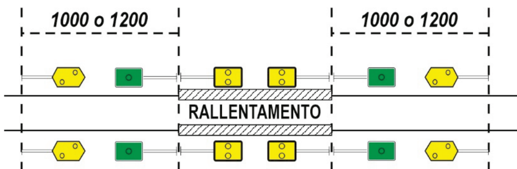
Rallentamento su linea a doppio binario interessando ambedue i binari
