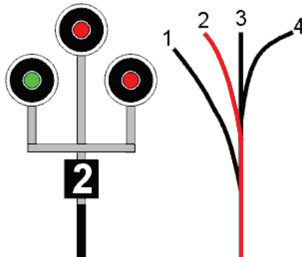
Segnale a candelieri integrato da indicatore a via libera per la direzione 2.
